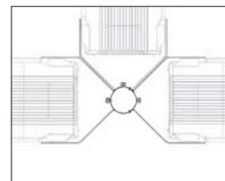
Mastaufsatz für 3 Scheinwerfer 90° ohne Bügel \varnothing 102 mm, L: 750 mm Column top for 3 plane projector 90° without mounting bracket \varnothing 102 mm, L: 750 mm
