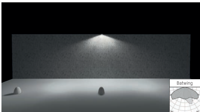
Batwing 150^\circ \times 15^\circ
