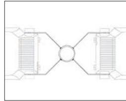
Mastaufsatz für 2 Scheinwerfer 180° ohne Bügel \varnothing 76 mm, L: 200 mm Column top for 2 plane projector 180° with-out mounting bracket \varnothing 76 mm, L: 200 mm
