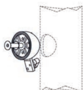
Mastansatzstück für seitliche Mast-anbindung in: \varnothing 60 mm; \varnothing 76 mm; \varnothing 90 mm oder \varnothing 114 mm Pole attachment, for lateral mounting arm \varnothing 60 mm; \varnothing 76 mm; \varnothing 90 mm or \varnothing 114 mm
