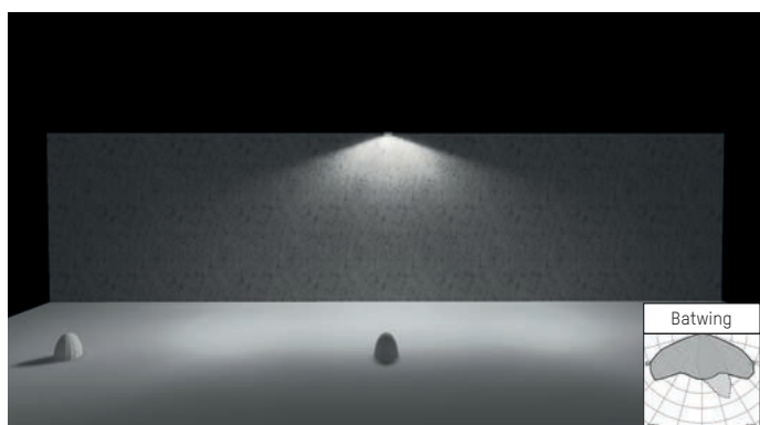
Batwing 150^\circ \times 15^\circ
