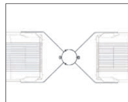
Mastaufsatz für 2 Scheinwerfer 180° ohne Bügel \varnothing 102 mm, L: 750 mm Column top for 2 plane projector 180° without mounting bracket \varnothing 102 mm, L: 750 mm
