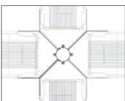
Mastaufsatz für 4 Scheinwerfer 90° ohne Bügel \varnothing 102 mm, L: 750 mm Column top for 4 plane projector 90° without mounting bracket \varnothing 102 mm, L: 750 mm
