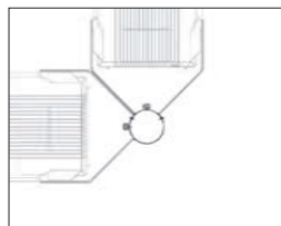
Mastaufsatz für 2 Scheinwerfer 90° ohne Bügel \varnothing 102 mm, L: 750 mm Column top for 2 plane projector 90° without mounting bracket \varnothing 102 mm, L: 750 mm
