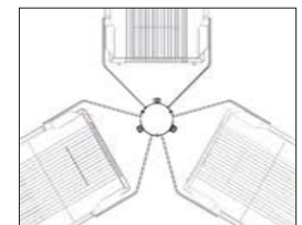
Mastaufsatz für 3 Scheinwerfer 120° ohne Bügel \varnothing 102 mm, L: 750 mm Column top for 3 plane projector 120° without mounting bracket \varnothing 102 mm, L: 750 mm
