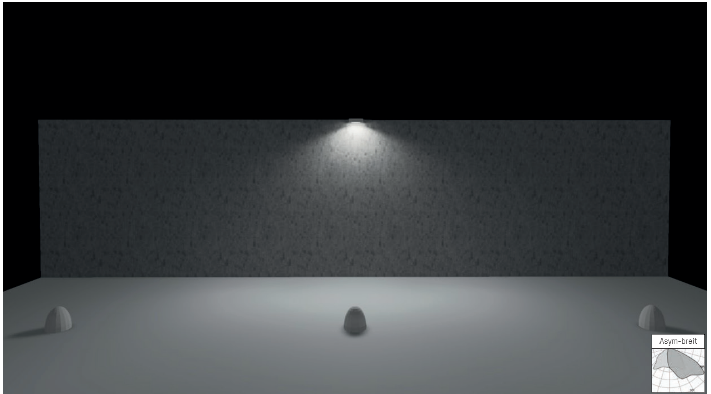
Asymmetrisch breitstrahlend 125° x 45°
