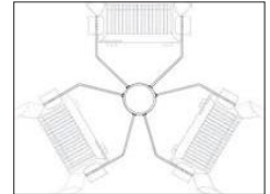
Mastaufsatz für 3 Scheinwerfer 120° ohne Bügel \varnothing 76 mm, L: 200 mm Column top for 3 plane projector 120° with-out mounting bracket \varnothing 76 mm, L: 200 mm
