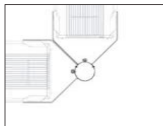
Mastaufsatz für 2 Scheinwerfer 90° ohne Bügel \varnothing 102 mm, L: 750 mm Column top for 2 plane projector 90° without mounting bracket \varnothing 102 mm, L: 750 mm
