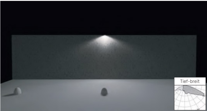
Tief-breitstrahlend 125° x 67°
