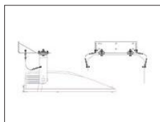
Wandhalter, Erschütterungsgedämpft Wall bracket, anti-vibration mounting
