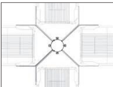
Mastaufsatz für 4 Scheinwerfer 90° ohne Bügel \varnothing 102 mm, L: 750 mm Column top for 4 plane projector 90° without mounting bracket \varnothing 102 mm, L: 750 mm
