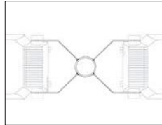
Mastaufsatz für 2 Scheinwerfer 180° ohne Bügel \varnothing 76 mm, L: 200 mm Column top for 2 plane projector 180° with-out mounting bracket \varnothing 76 mm, L: 200 mm
