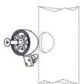
Mastansatzstück für seitliche Mast- anbindung in: \phi 60 mm; \phi 76 mm; \phi 90 mm oder \phi 114 mm Pole attachment, for lateral moun- ting arm \phi 60 mm; \phi 76 mm; \phi 90 mm or \phi 114 mm
