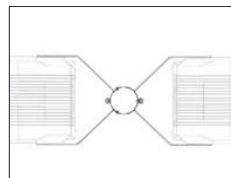
Mastaufsatz für 2 Scheinwerfer 180° ohne Bügel \varnothing 102 mm, L: 750 mm Column top for 2 plane projector 180° without mounting bracket \varnothing 102 mm, L: 750 mm
