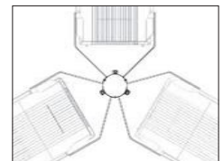
Mastaufsatz für 3 Scheinwerfer 120° ohne Bügel \varnothing 102 mm, L: 750 mm Column top for 3 plane projector 120° without mounting bracket \varnothing 102 mm, L: 750 mm
