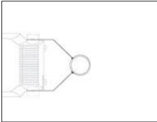
Mastaufsatz für 1 Scheinwerfer ohne Bügel \varnothing 76 mm, L: 200 mm Column top for 1 plane projector with-out mounting bracket \varnothing 76 mm, L: 200 mm
