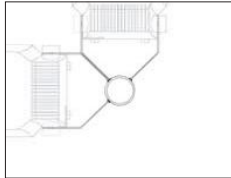
Mastaufsatz für 2 Scheinwerfer 90° ohne Bügel \varnothing 76 mm, L: 200 mm Column top for 2 plane projector 90° with-out mounting bracket \varnothing 76 mm, L: 200 mm
