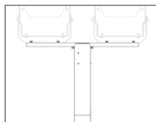
Traversenaufsatz für zwei 155er mit Mastdurchmesser 102 mm, L: 750 mm Traverse attachment, for two 155 with column diameter 102 mm, L: 750 mm
