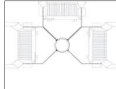
Mastaufsatz für 3 Scheinwerfer 90° ohne Bügel \varnothing 76 mm, L: 200 mm Column top for 3 plane projector 90° with-out mounting bracket \varnothing 76 mm, L: 200 mm
